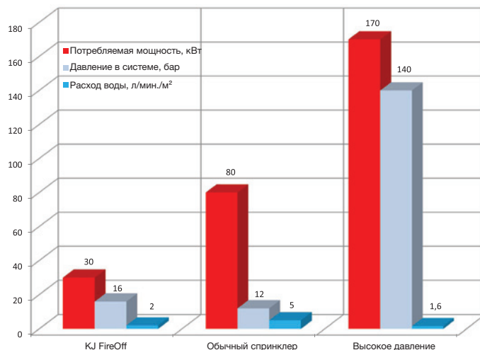
СРАВНЕНИЕ СИСТЕМЫ ОГНЕТУШЕНИЯ С ИСПОЛЬЗОВАНИЕМ ТОНКОРАСПЫЛЕННОЙ ВОДЫ И СТАНДАРТНОЙ СПРИНКЛЕРНОЙ СИСТЕМЫ
